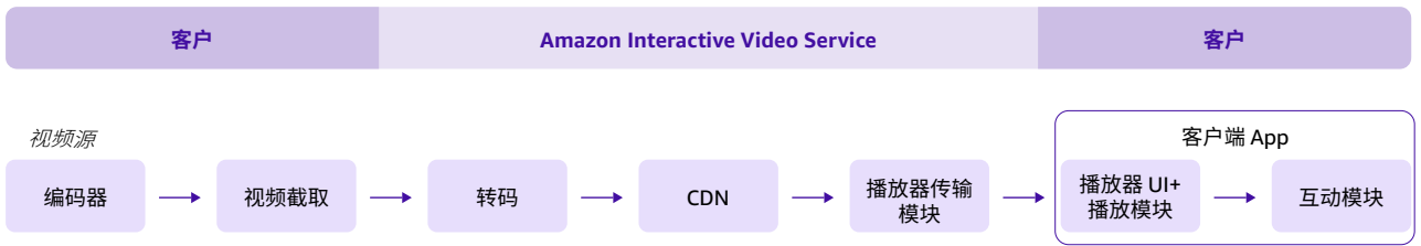
图 17 直播短视频互动解决方案示意
